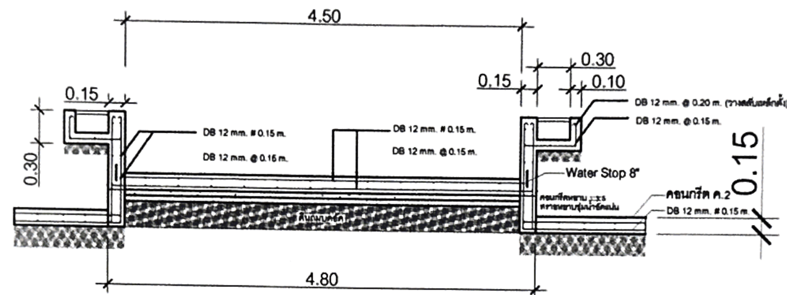
แบบแสดงแนวตัด C-C 1:50
