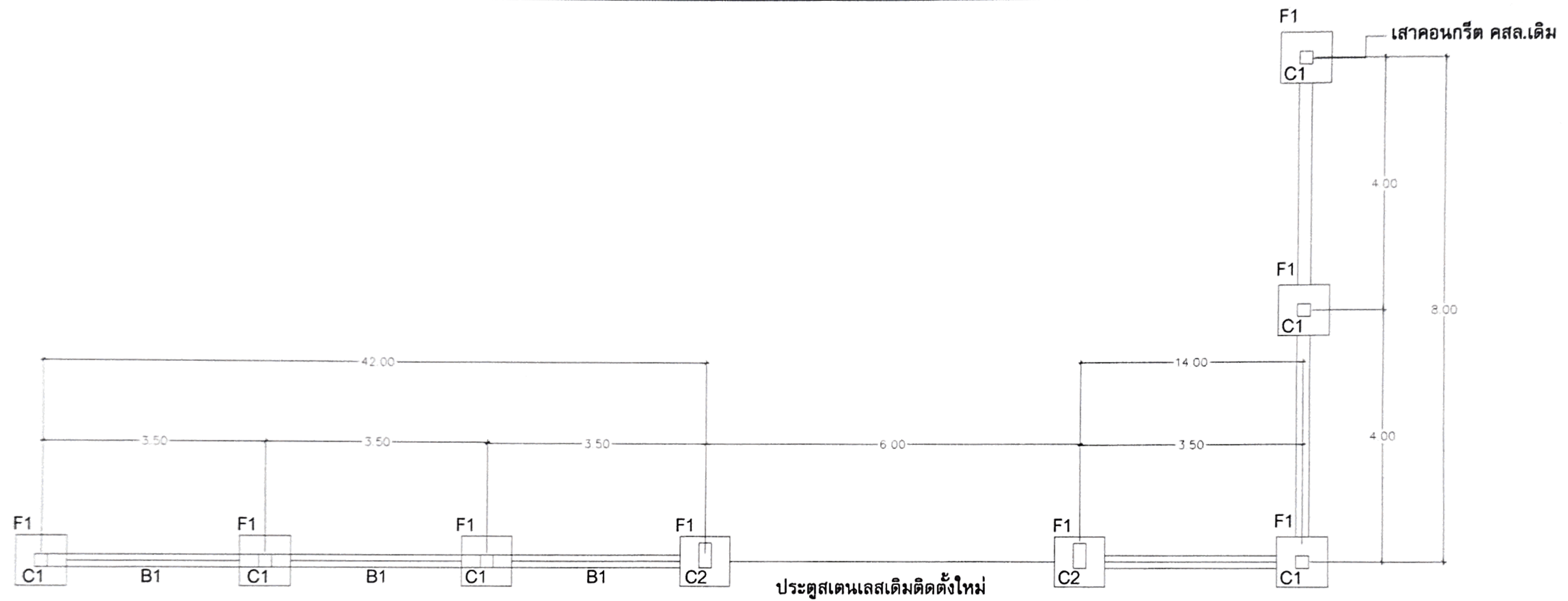
แปลนฐานราก คาน เสา SCALE 1:150
