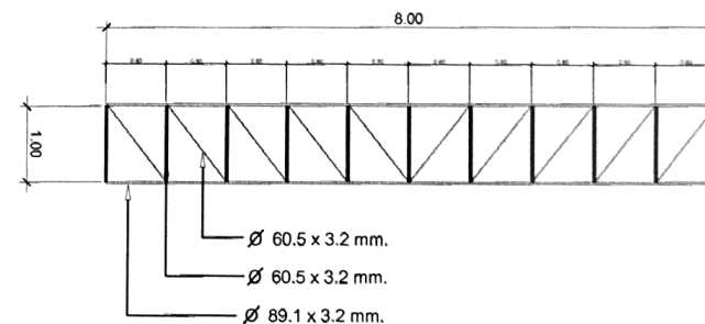
แบบขยาย TRUSS B
